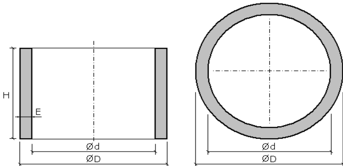
ARO PARA POZO
