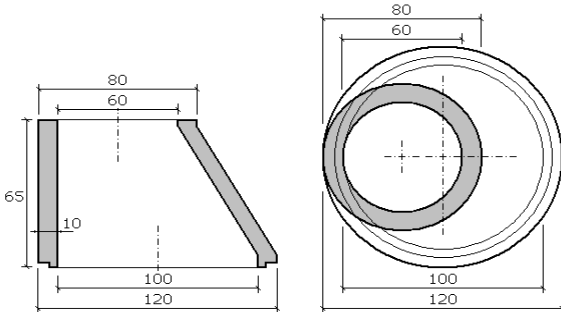
MODULO CONICO ASIMETRICO PARA POZO - REDUCCION DE Ø 100 cm a Ø 60 cm.
