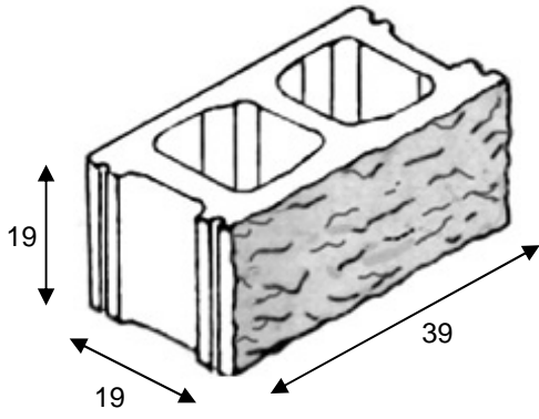
Bloque SPLIT Estándar 39 x 19 x 19
