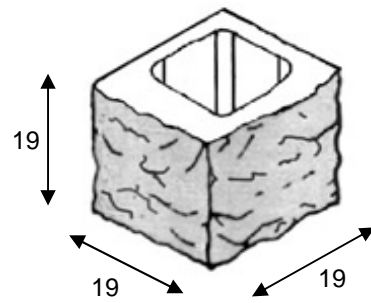
Medio SPLIT Esquina 19 x 19 x 19
