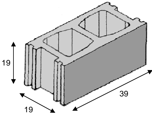
Bloque LISO Estándar 39 x 19 x 19
